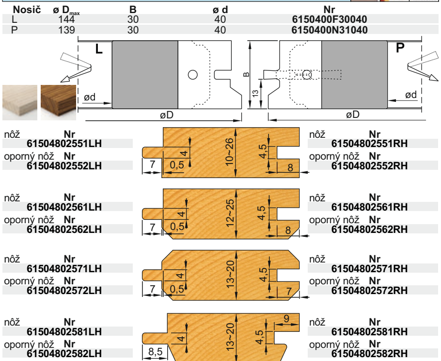
Univerzálny systém fréz pre profily typu pero-drážka. Nosiče sa osádzajú vybraným typom nôžov.
