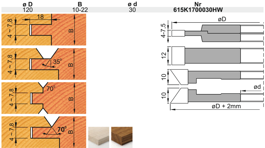
Remeselná sada fréz pre štyri druhy profilov pero-drážky.
