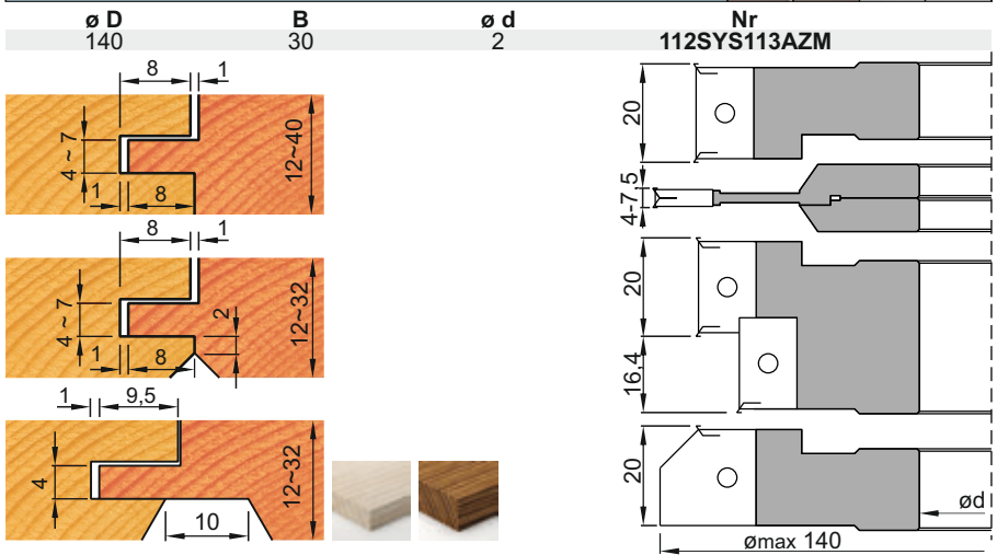
Sada pozostávajúca zo 4 nástrojov, kombináciou ktorých je možné dosiahnuť 3 typy profilov. Nástroje sú určené pre spodné frézovačky a sú vhodné aj pre ručný posuv.
