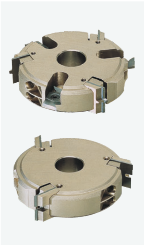
Univerzálny systém fréz pre profily typu pero-drážka. Nosiče sa osádzajú vybraným typom nôžov.
