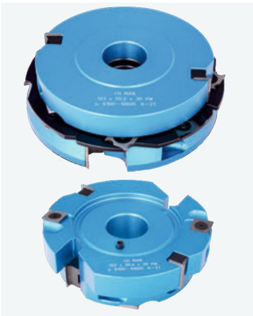
Sada pozostávajúca zo 4 nástrojov, kombináciou ktorých je možné dosiahnuť 3 typy profilov. Nástroje sú určené pre spodné frézovačky a sú vhodné aj pre ručný posuv.
